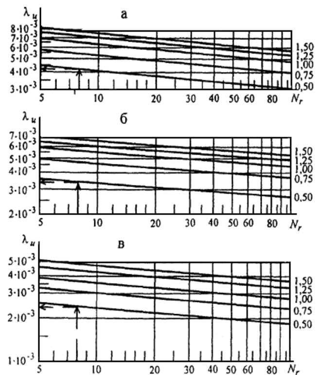
Рисунок К.4 - Номограмма для определения коэффициента \psi_k
