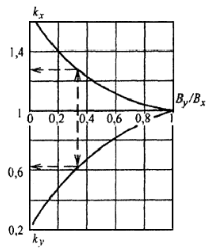
Рисунок К.1 - Значения переходных коэффициентов k
