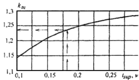
Рисунок К.2 - График для определения коэффициентов k_x и k_y , учитывающих перераспределение внутренних усилий в ортотропных плитах
