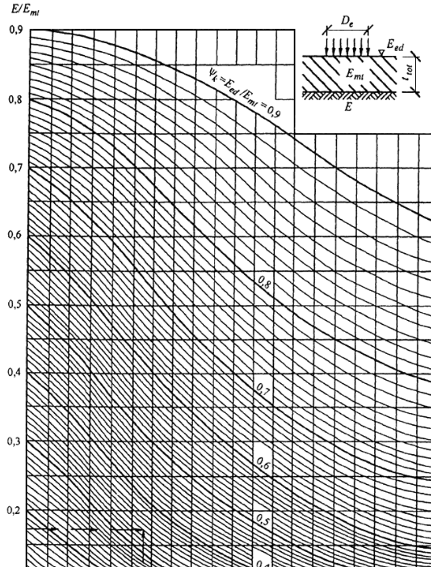
Рисунок К.3 - График для определения поправочного коэффициента k_m при расчете толщины усиления бетонного покрытия
