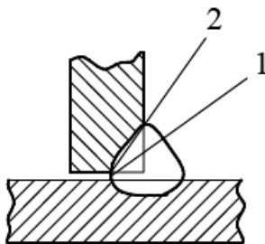
1 - по металлу шва; 2 - по металлу границы сплавления
