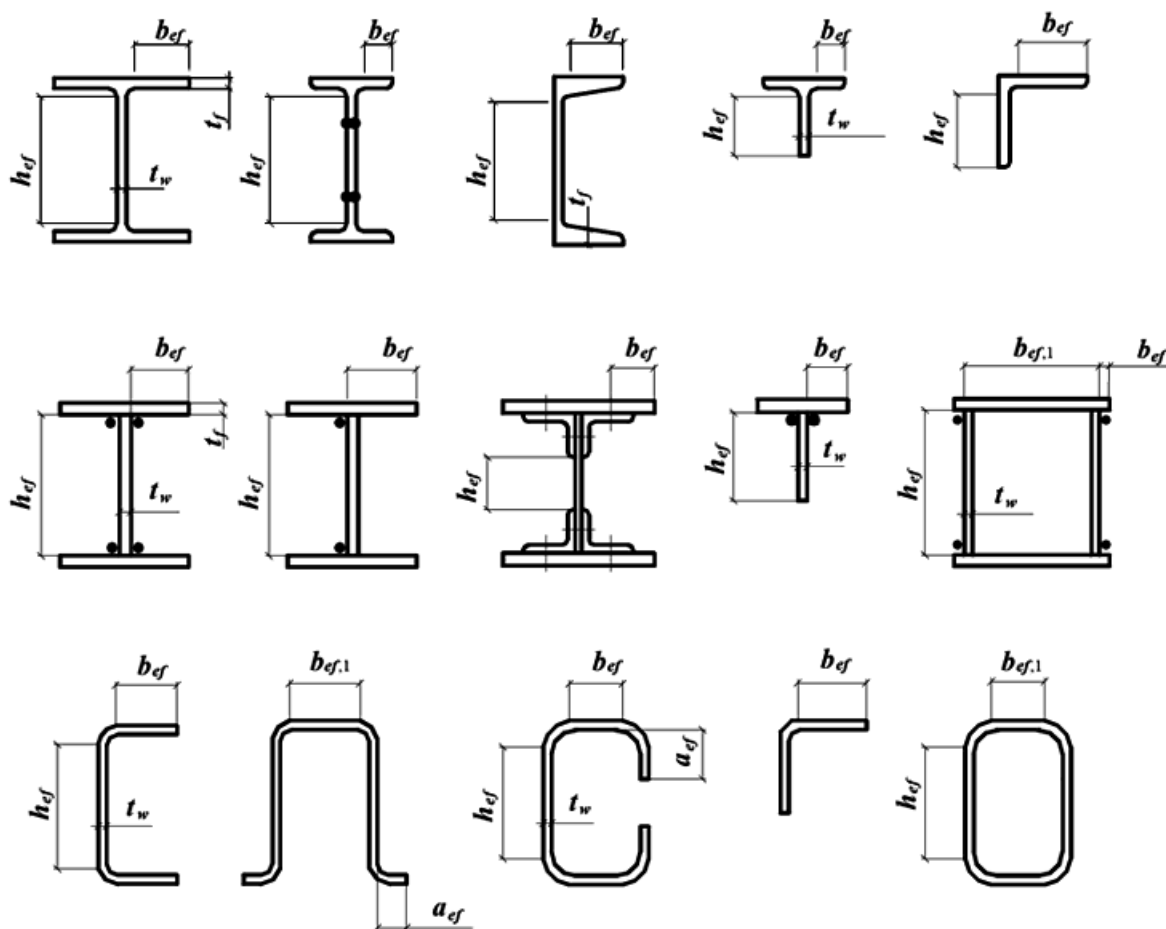
Рисунок 5 - Расчетные размеры стенок, свесов полков, поясных листов в прокатных, составных и гнутых профилях полную высоту стенки - в сварных элементах;
