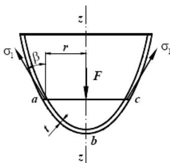
Рисунок 16 - Схема оболочки вращения
