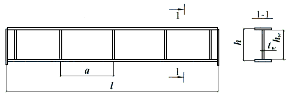
Рисунок М.1 - Схема балки с гибкой стенкой
