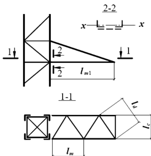
Рисунок 22 - Схема траверсы с треугольной решеткой
