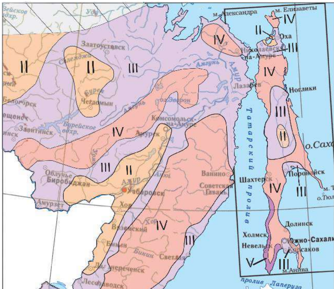
КАРТА 3, в. РАЙОНИРОВАНИЕ ТЕРРИТОРИИ ПРИМОРСКОГО КРАЯ И ОСТРОВА САХАЛИН ПО ТОЛЩИНЕ СТЕНКИ ГОЛОЛЁДА
