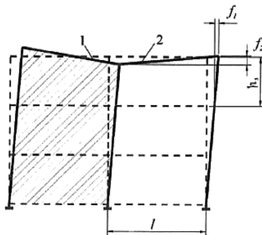
Рисунок Д.2 - Схема для определения прогибов стропильных конструкций при наличии подвесных крановых путей
