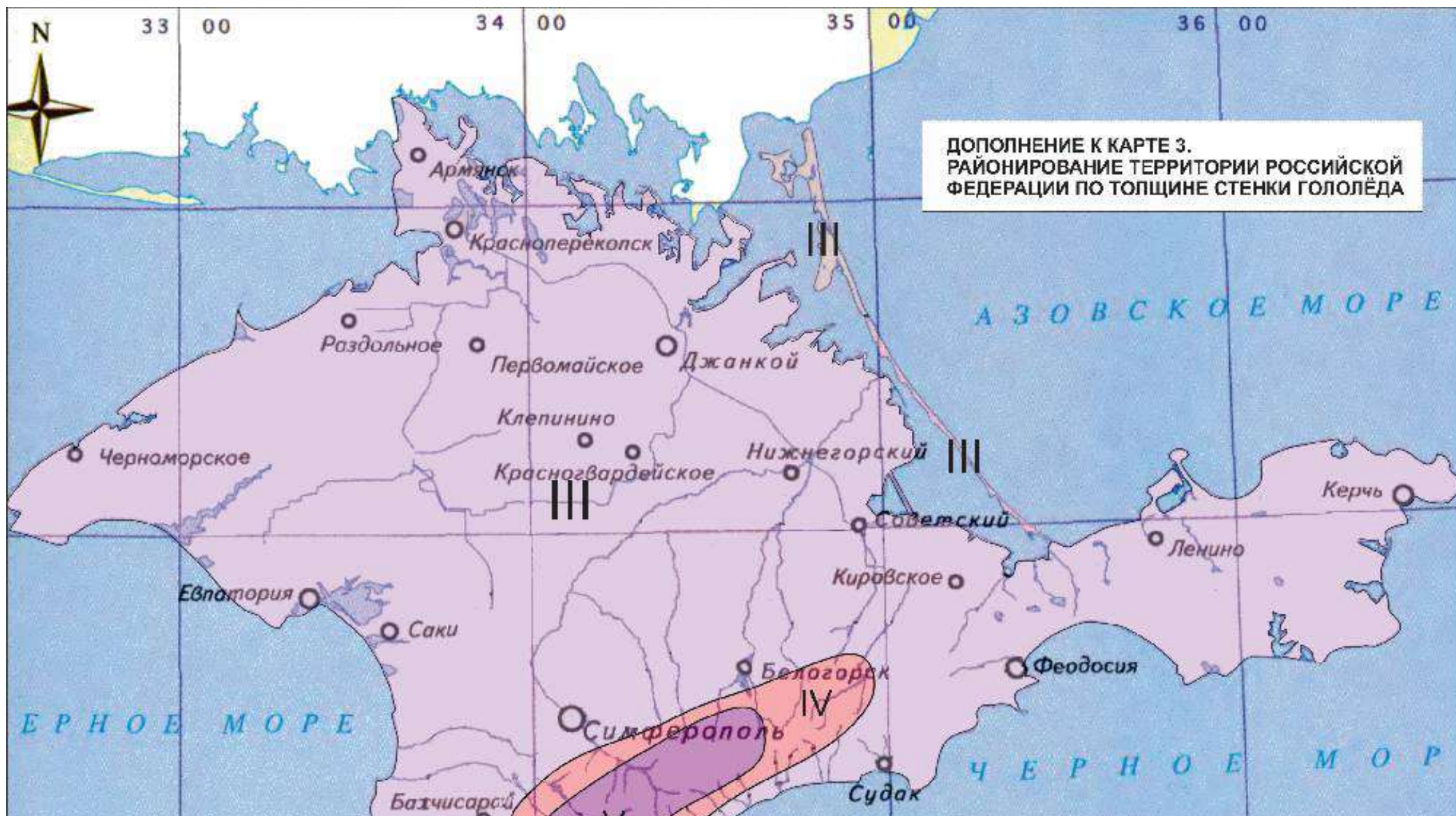
КАРТА 3, 6. РАЙОНИРОВАНИЕ ТЕРРИТОРИИ РЕСПУБЛИКИ КРЫМ ПО ТОЛЩИНЕ СТЕНКИ ГОЛОЛЁДА
