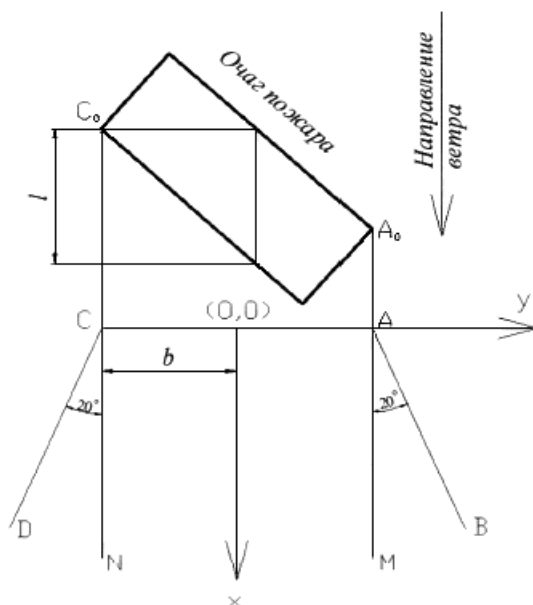
Рисунок Е.2 - Схема определения размеров зон загазованности от отдельного очага пожара при направлении ветра под острым углом к фасаду здания
