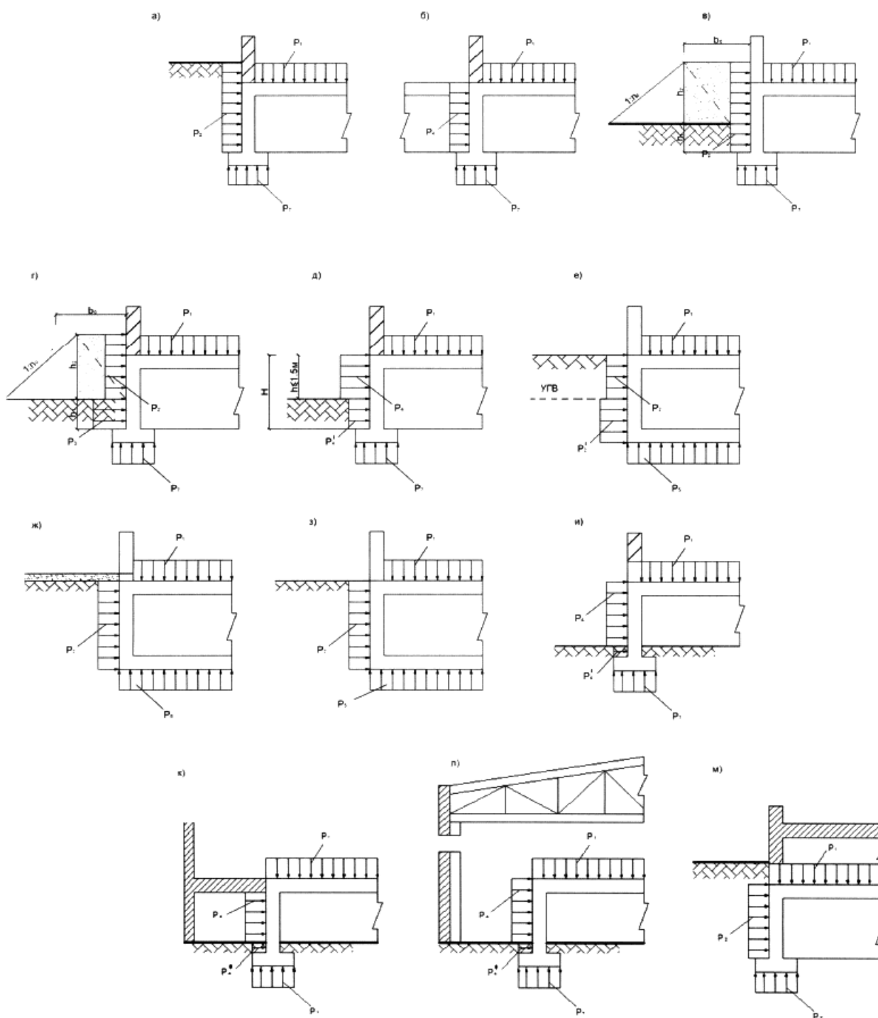
Рисунок 7.1 - Схемы приложения динамических нагрузок на конструкции убежищ
